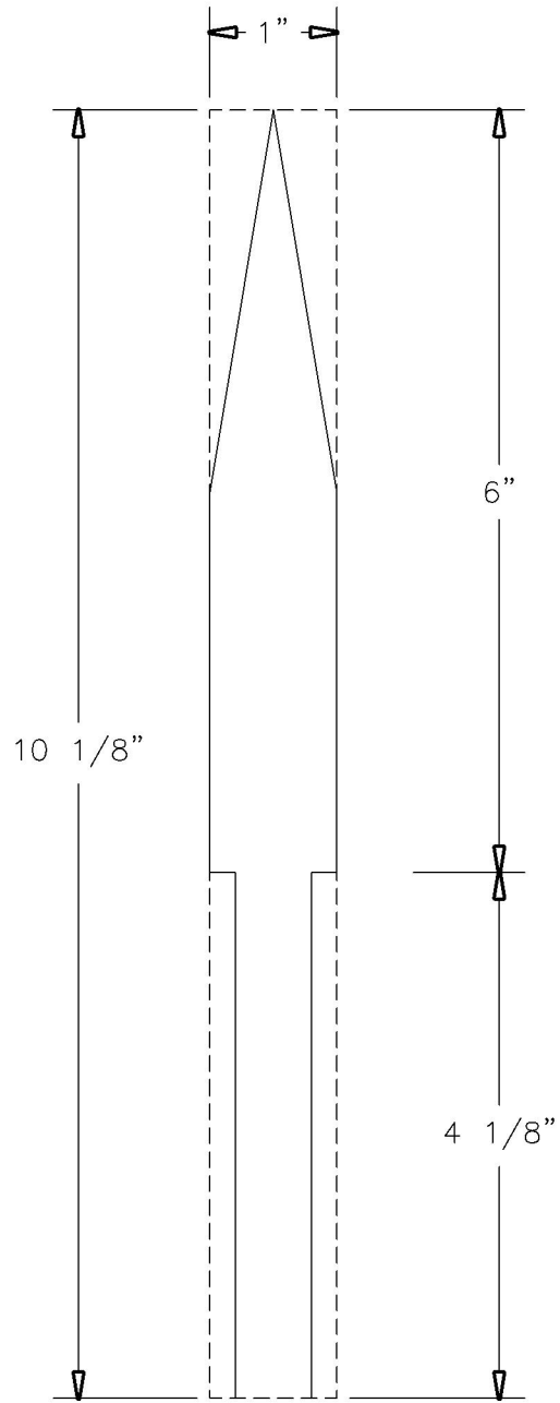
Blade
