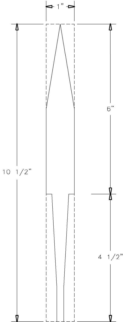
Blade
